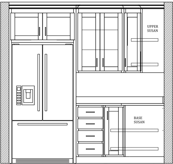
1 ELEVATION A1.01 SCALE: .
