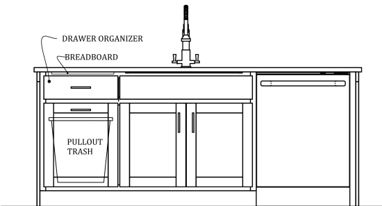
3 ELEVATION A1.01 SCALE: .
