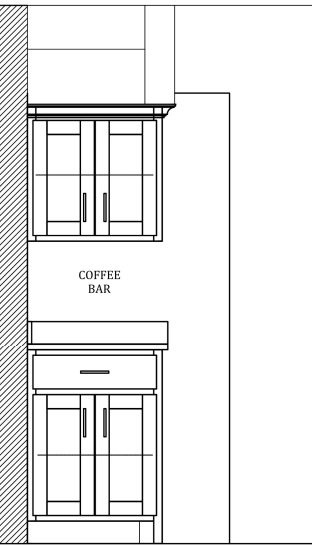
4 ELEVATION A1.01 SCALE: .
